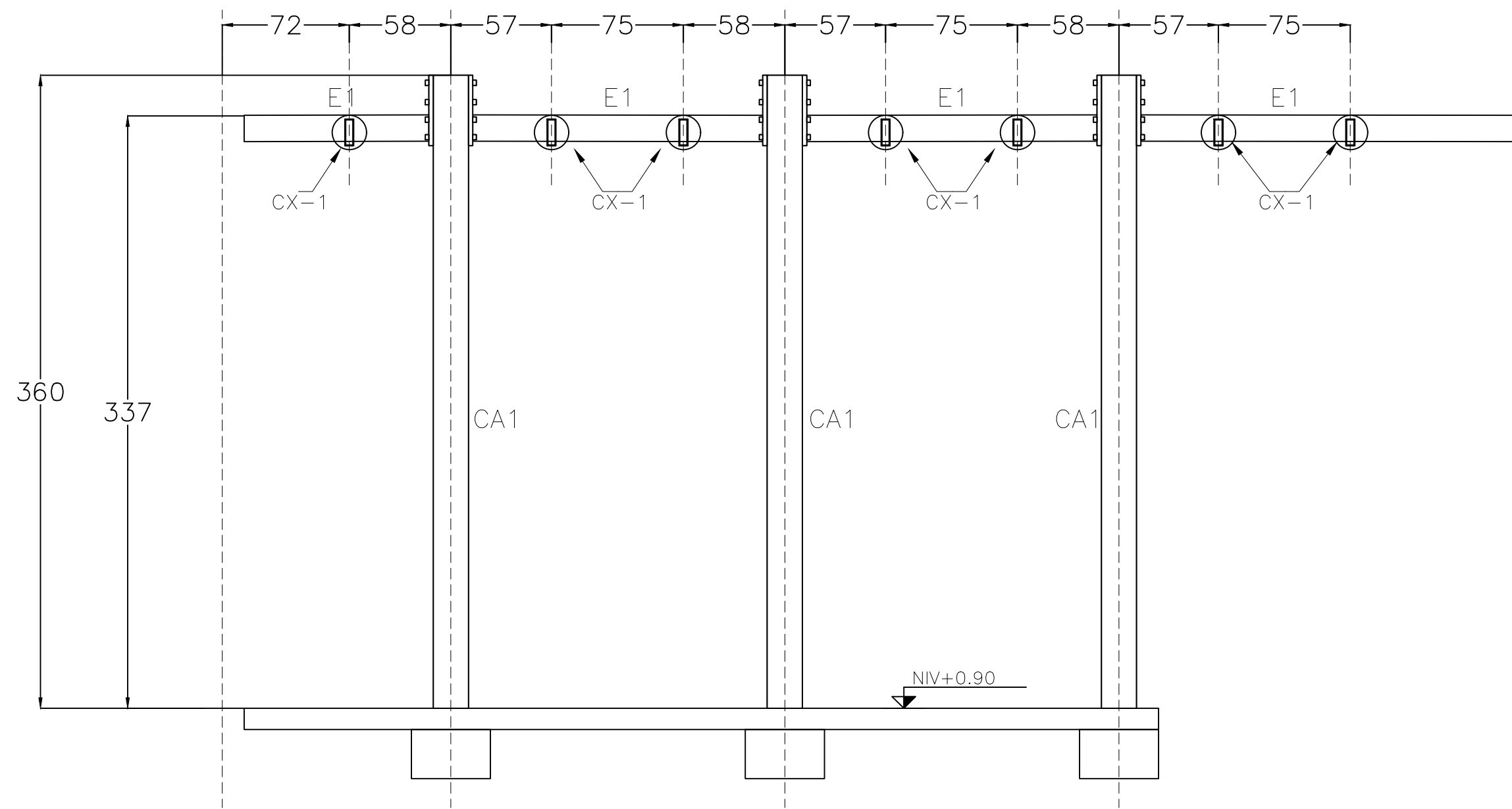
MARCO LONGITUDINAL CUBIERTA 2 Acot: mm
