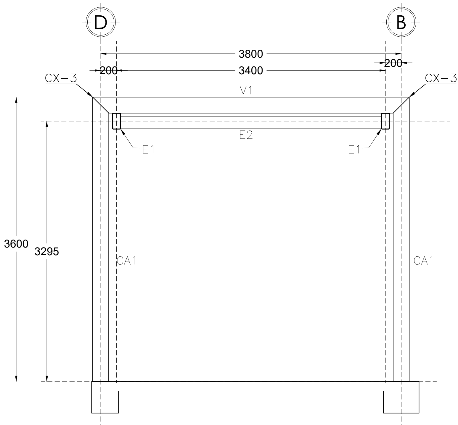
MARCO TRANSVERSAL CUBIERTA 2 Acot: mm
