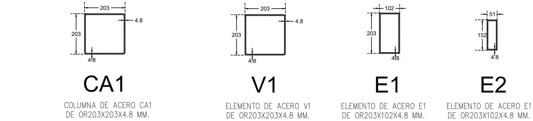
DETALLE COLUMNA CA1 Acot: mm DETALLE ELEMENTOS CUBIERTA Acot: mm
