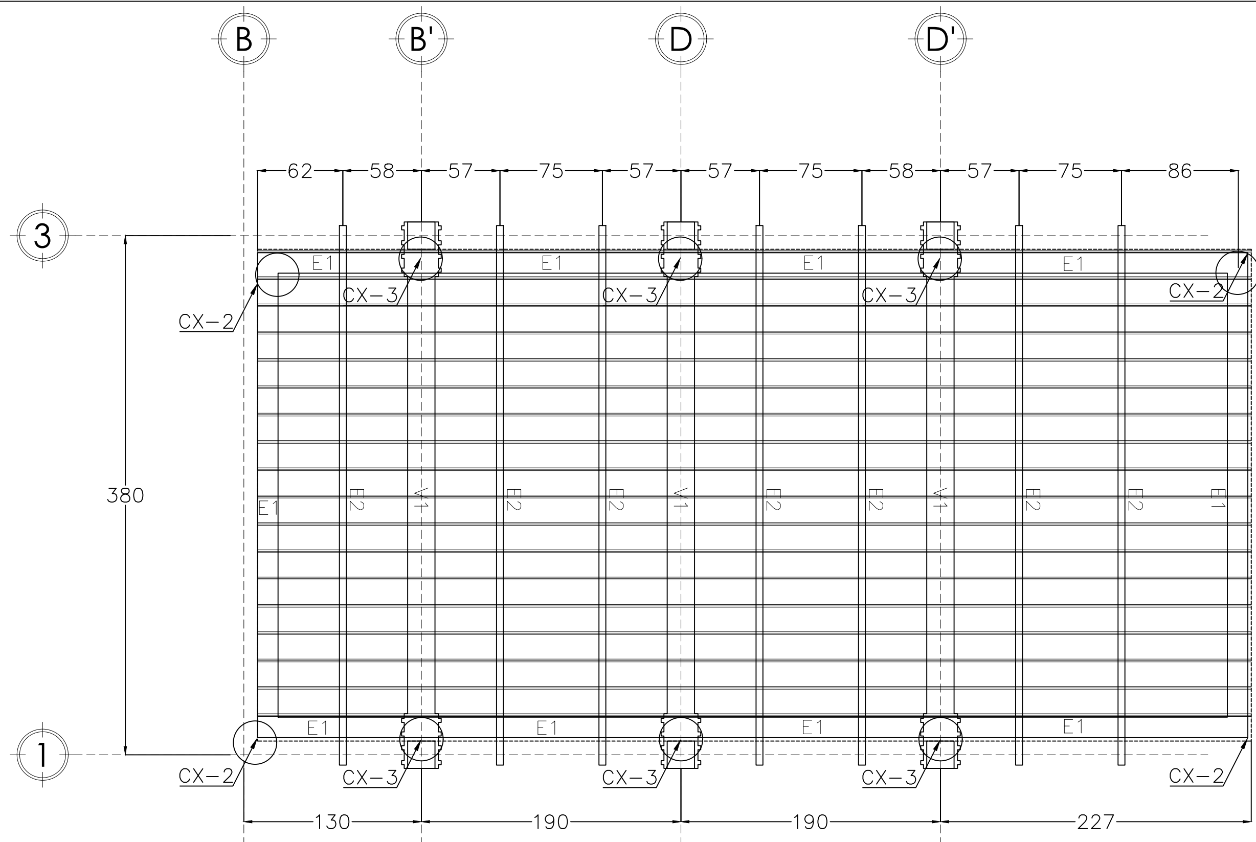
PLANTA DE CUBIERTA METÁLICA 2 Acot: mm
